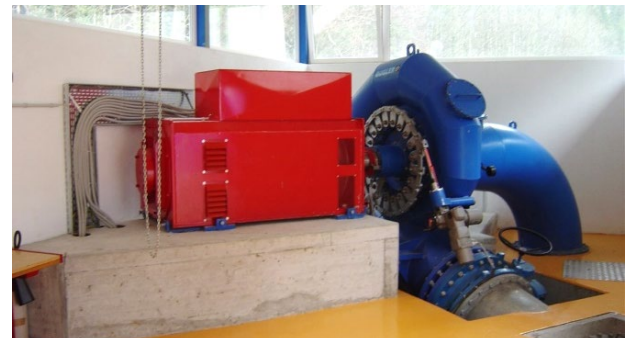
Spiral Francisturbine des Kraftwerks Blanches-Fontaines
